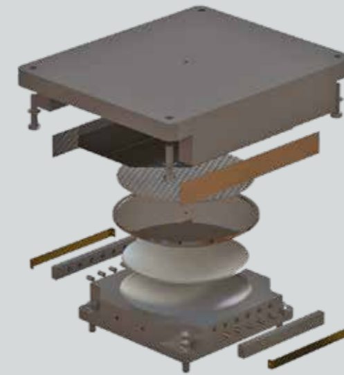
GE - Spherical (EN1337-7)
