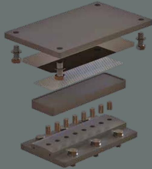
DE - Line Rocker (EN1337-6)
